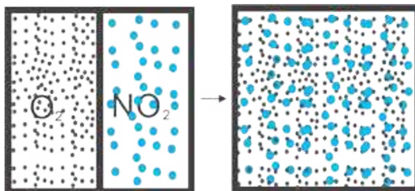
Fig (3.8) Diffusion
