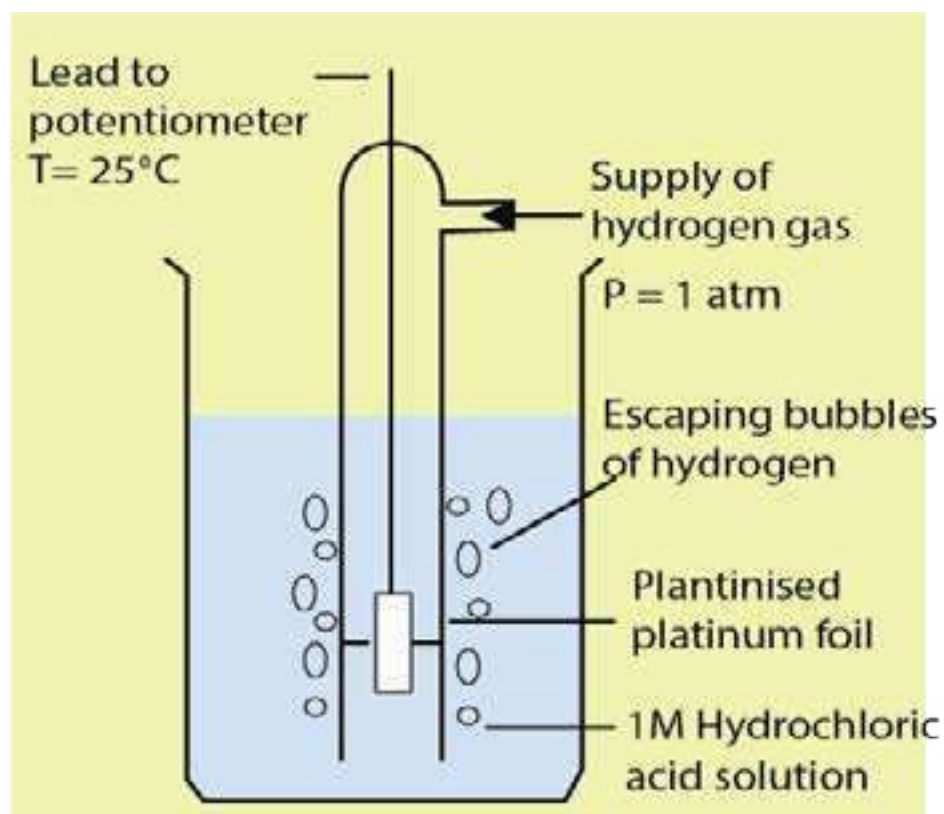
Fig.(10.4)Standardhydrogenelectrode(S.H.E)
