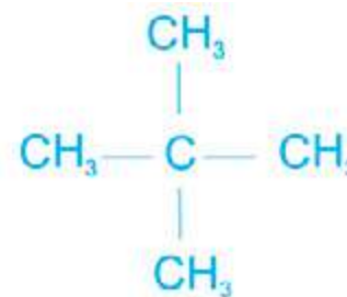
2,2 Dimethylpropane(neo-Pentane)
